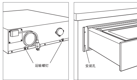
运输螺钉位置
